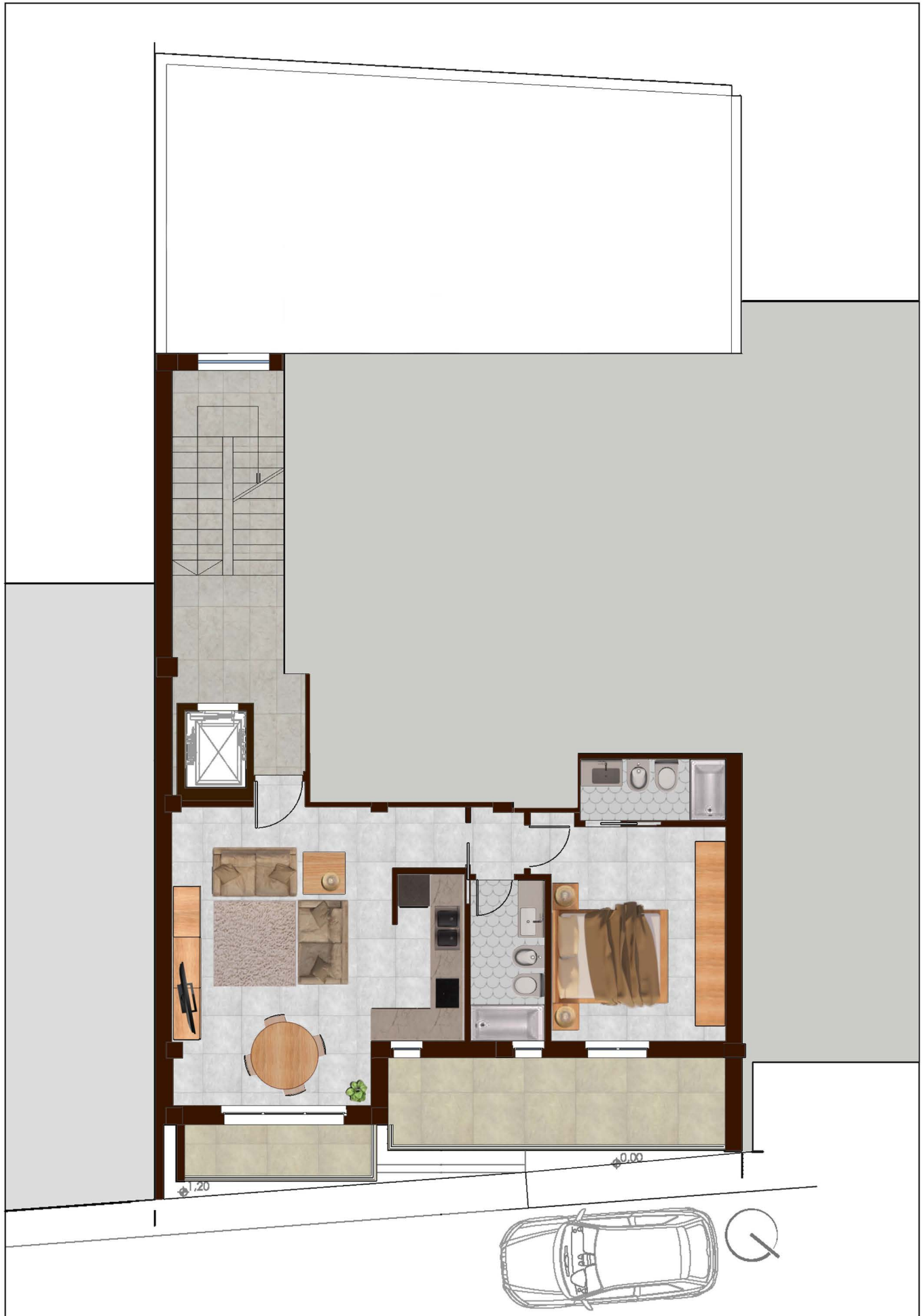
Abitazione 03 - piano primo - Scala 1:100
