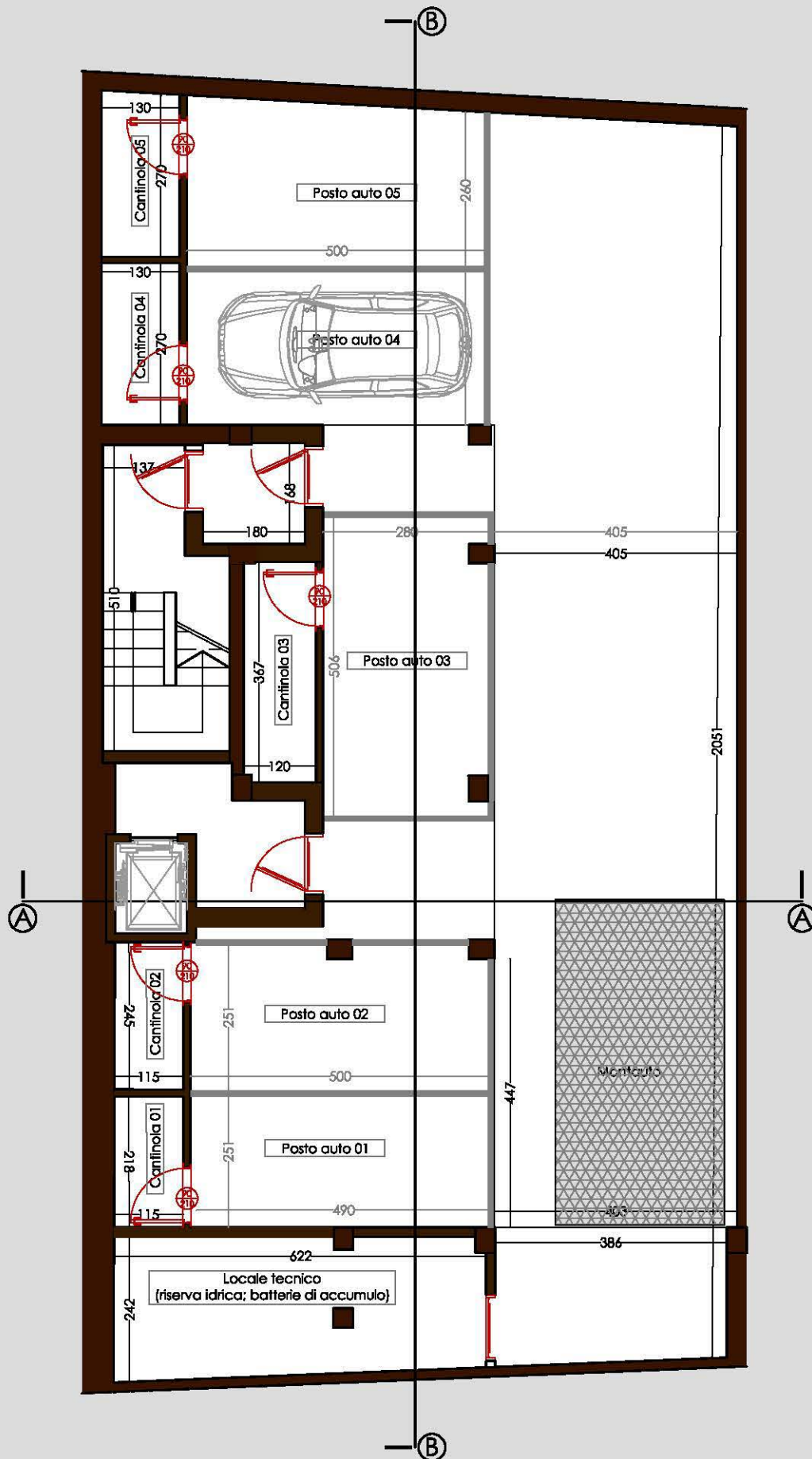
Planimetria piano interrato pertinenze abitazioni - Scala 1:100
